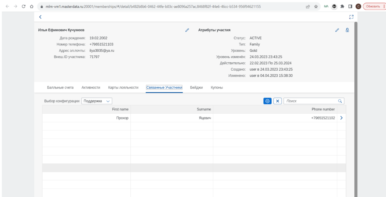
Рисунок 4.1.1.19. Внешний вид подраздела «Связанные участники» участника ПЭВМ «Masterdata Loyalty Management».
